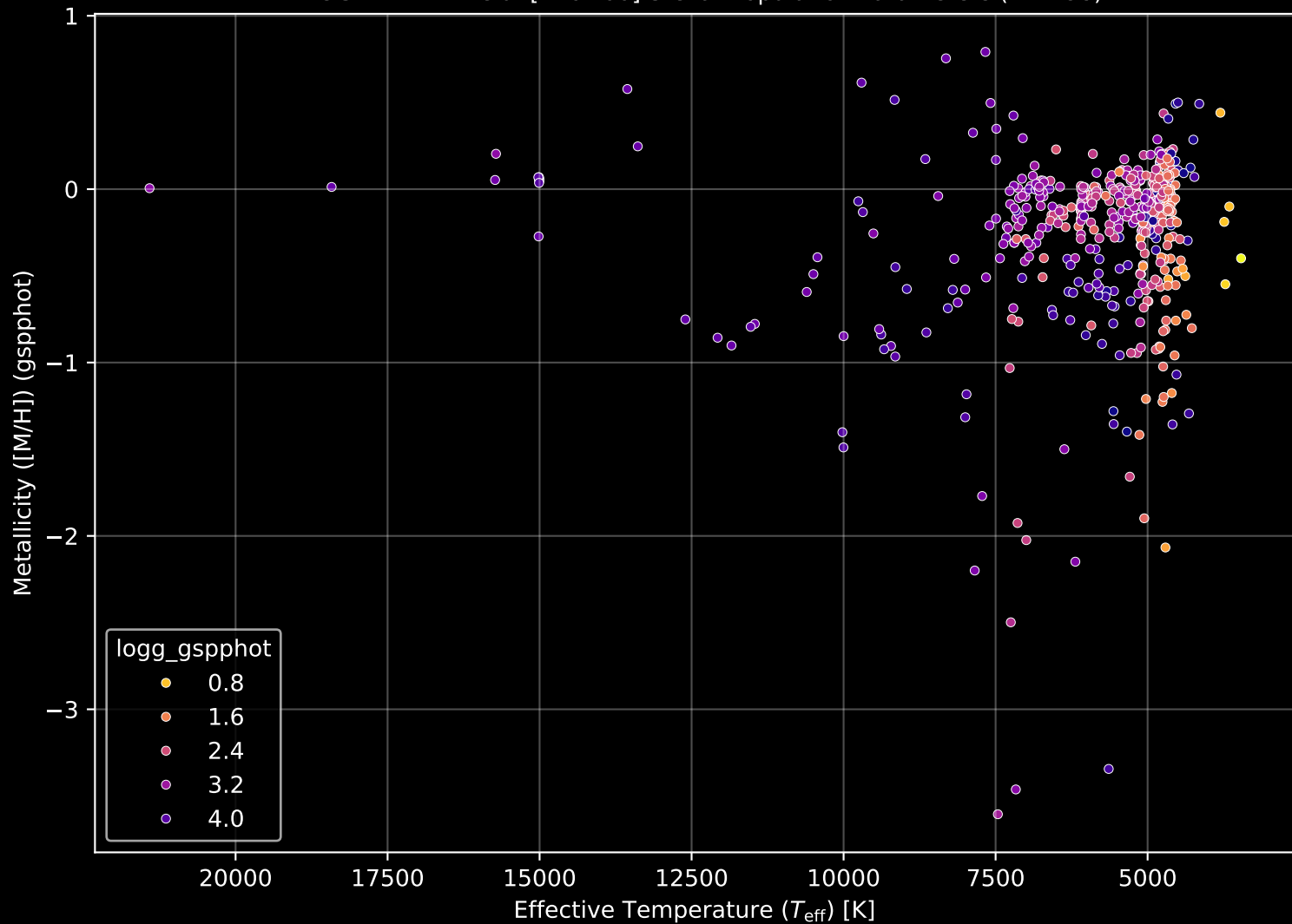
APOGEE DR17 Field: [176+00] Stellar Population Parameters (n= 498)
